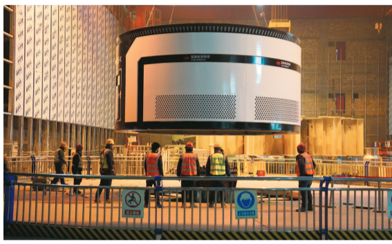
玛尔挡水电站首台(5号)发电机外罩安装。玛尔挡水电站供图
