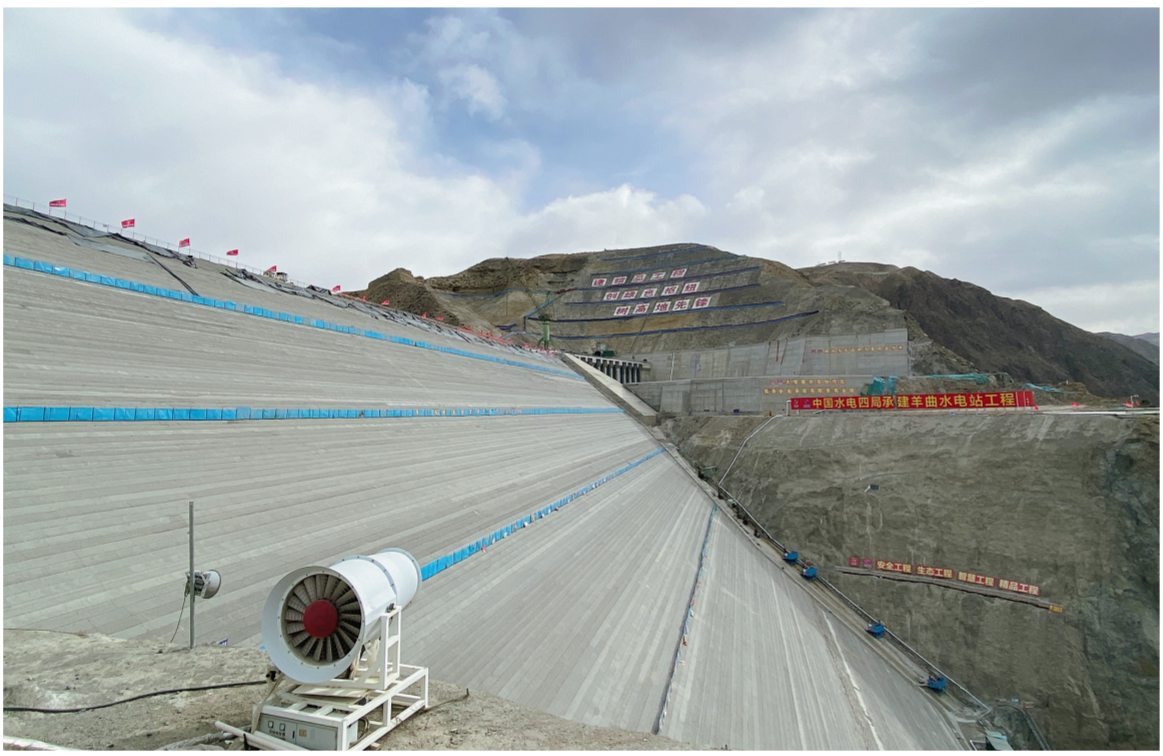
羊曲水电站大坝填筑施工完成。
