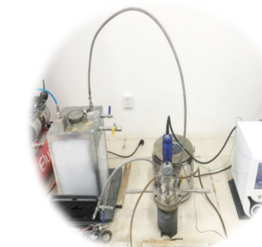
西宁麦戈帕沃科技有限公司的高效镁金属水解制氢装置。
